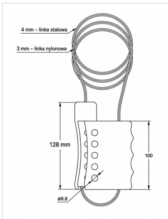
Blokowanie koła zaworu linką stalową.
