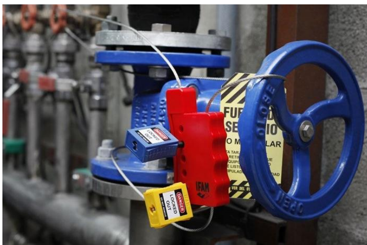
Blokowanie koła zaworu linką stalową.
